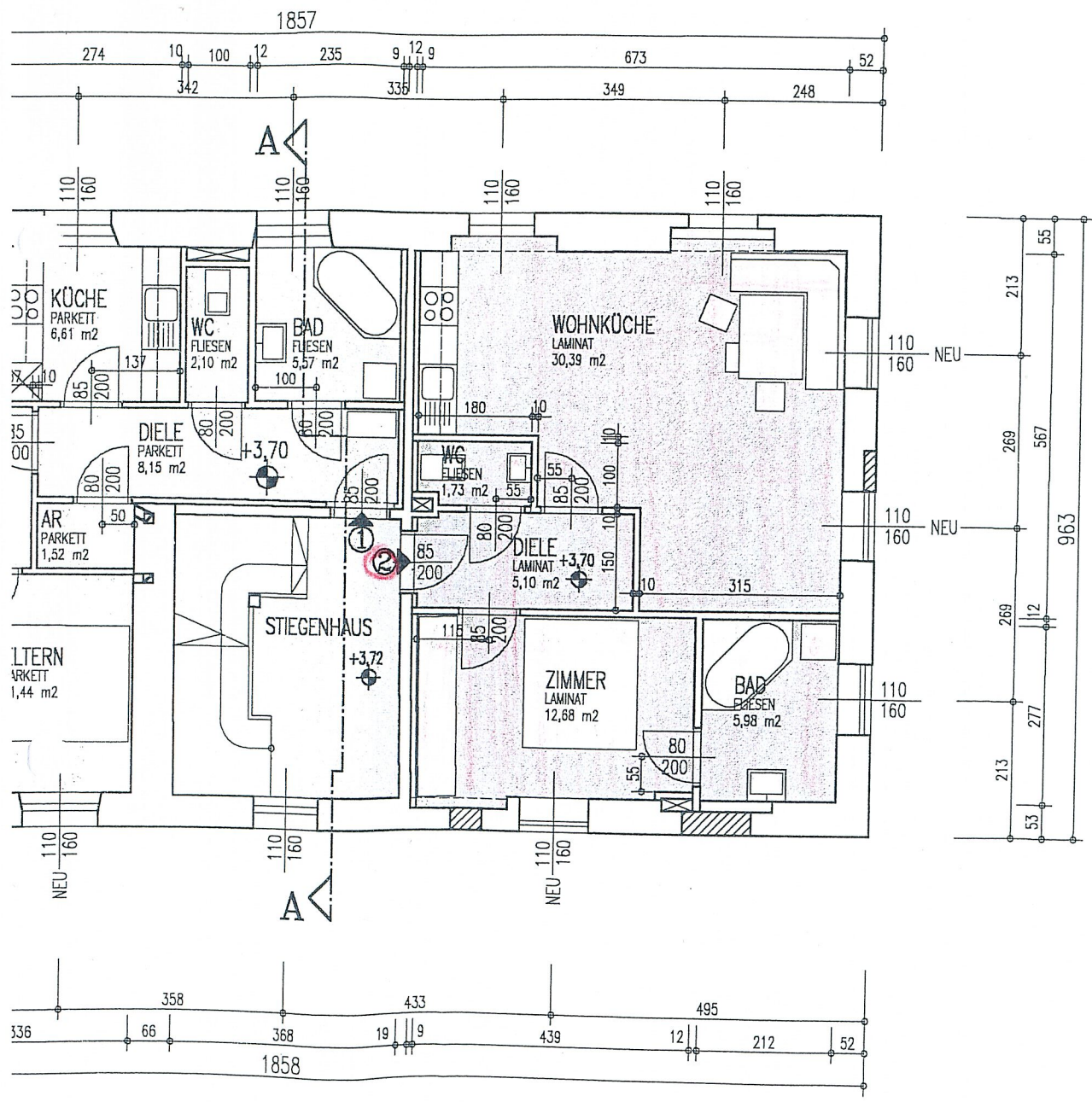
3. BERGESCHOSS M 1:100
